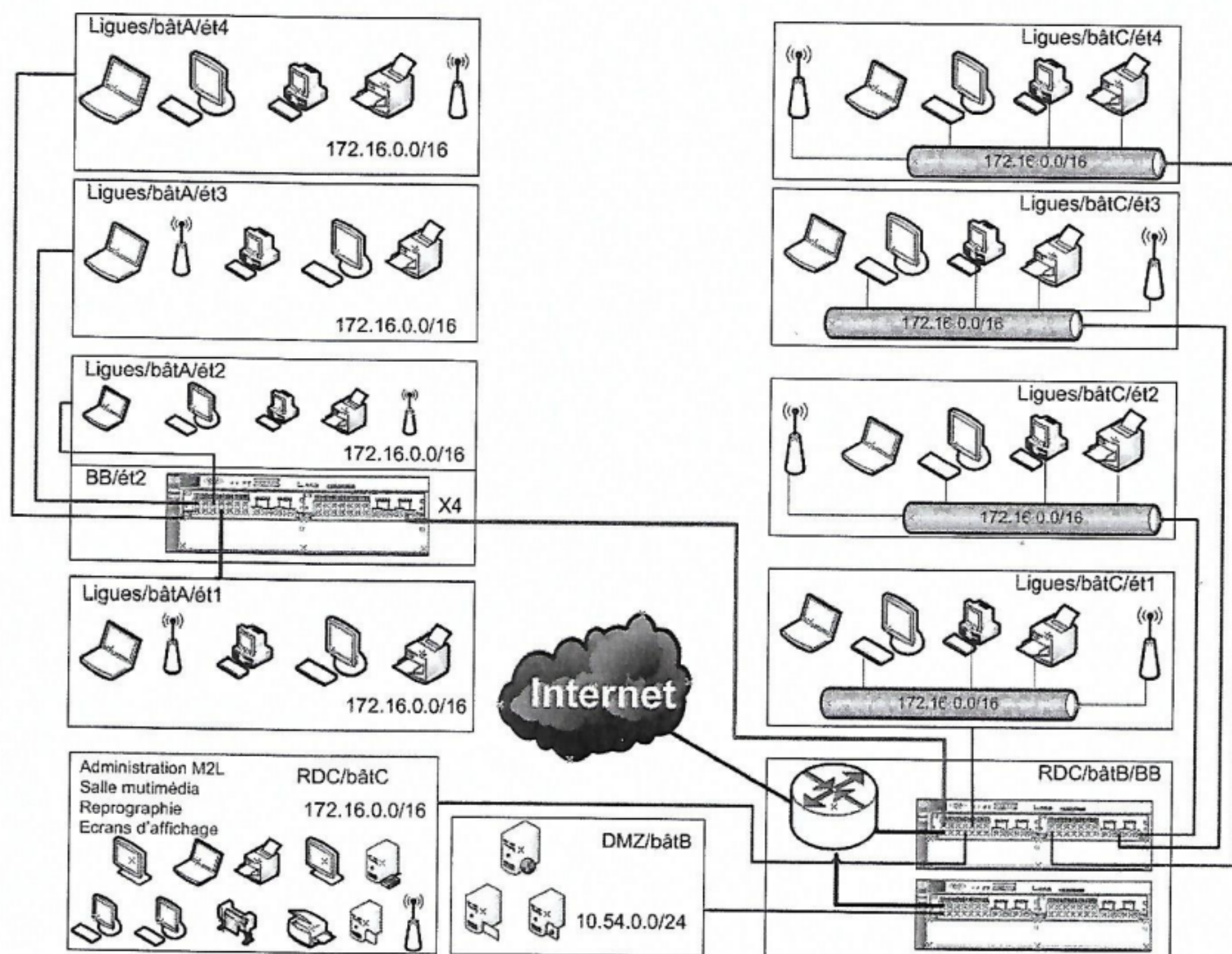
Schéma réseau
